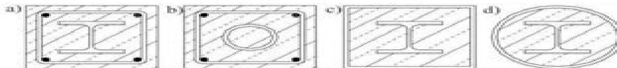
Fig. 4.9 - Composite Columns
